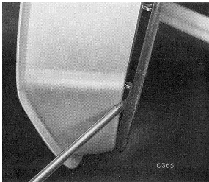
Fig. 30. Démontage du panneau de garniture de portière
