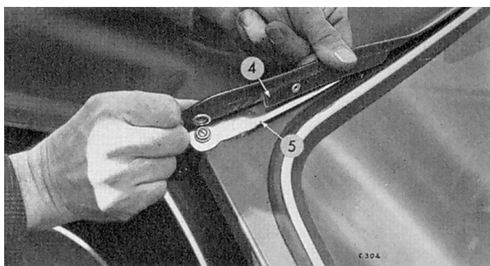
Fig. 44. Dégraissage de la partie avant de la capote
