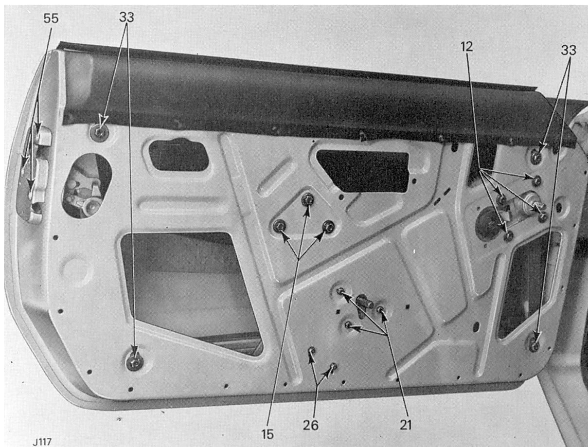
Fig. 34. Fixation des éléments de portière (Spitfire Mk. 2 et Mk. 3)
