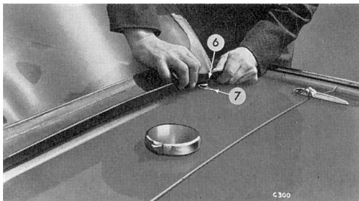
Fig. 45. Dégraissage de la partie arrière de la capote
