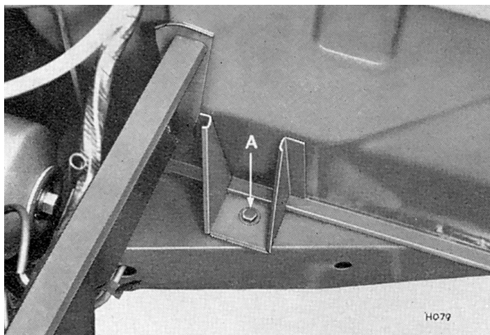
Fig. 2. Boulon de fixation du tablier à la traverse avant
