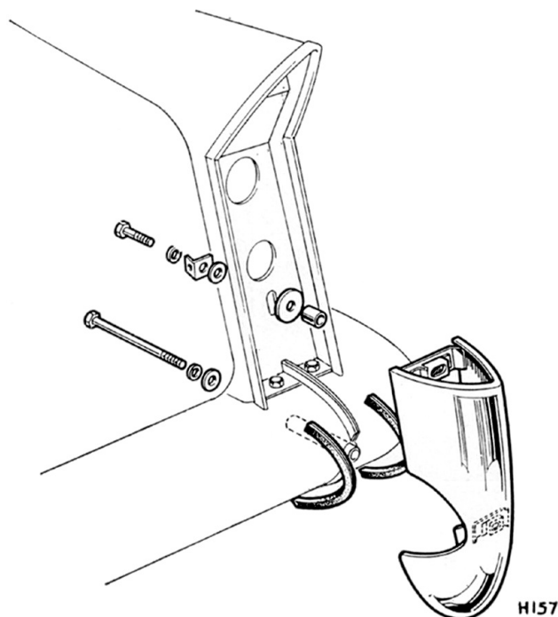
Fig. 20. Fixation de butoir arrière
