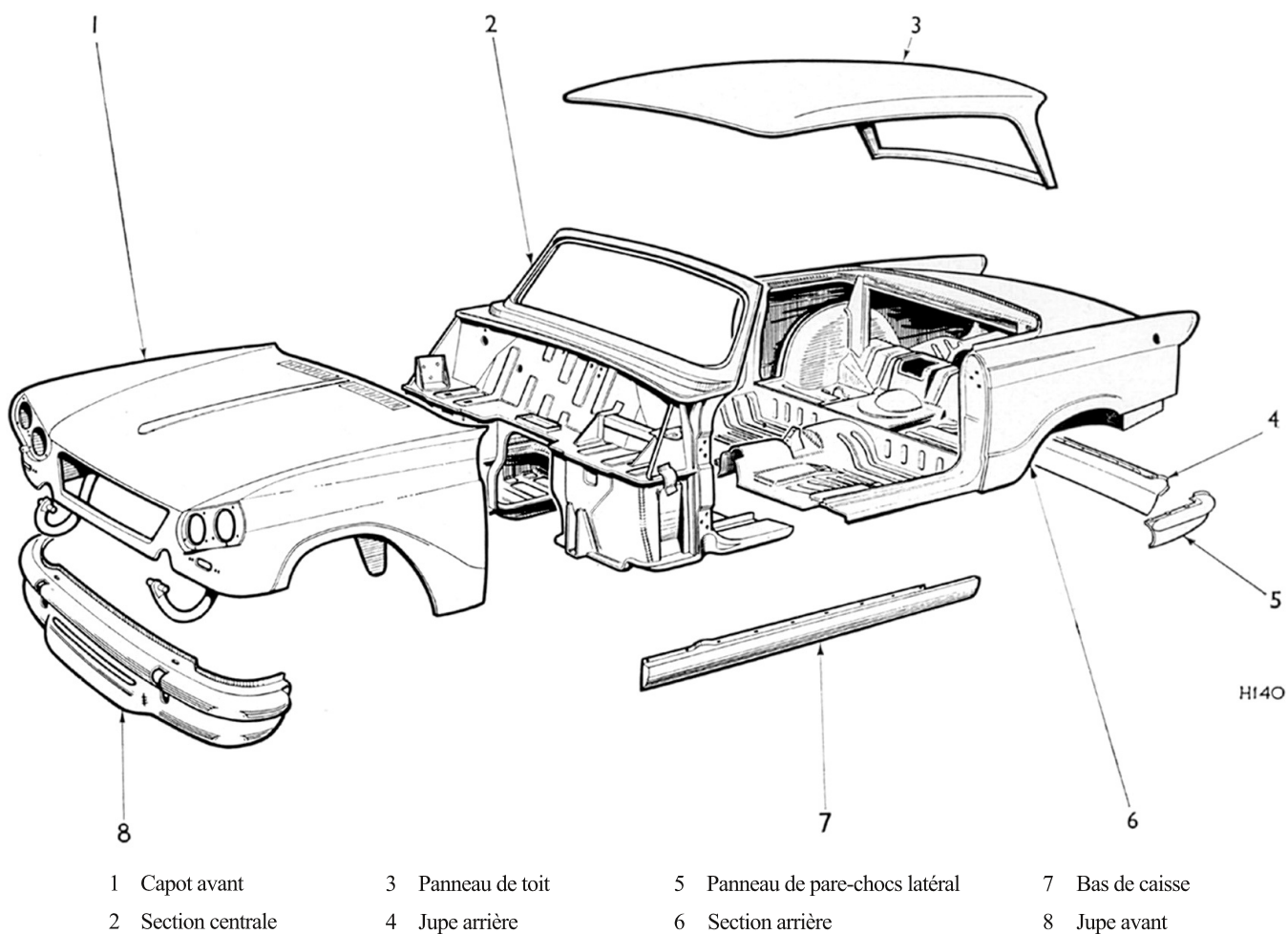
Fig. 7. Sous-ensembles de la carrosserie (Vitesse 6)
