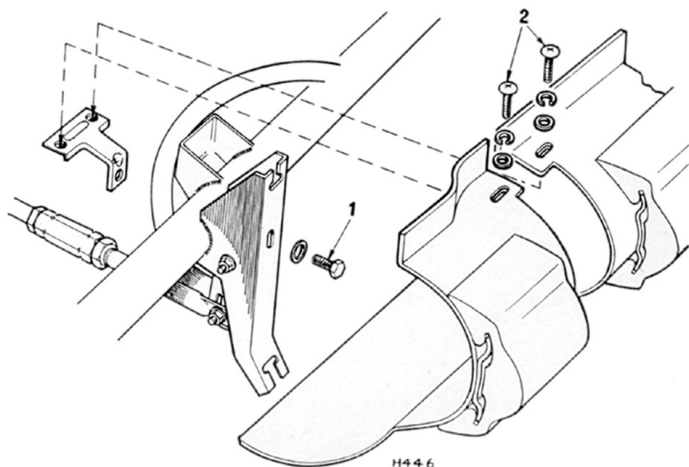
Fig. 18. Support de jupe avant
