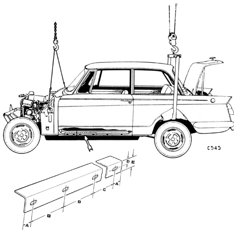
Fig. 6. Levage de la carrosserie (la flèche indique la position de la plaque de renfort du bas de caisse)
