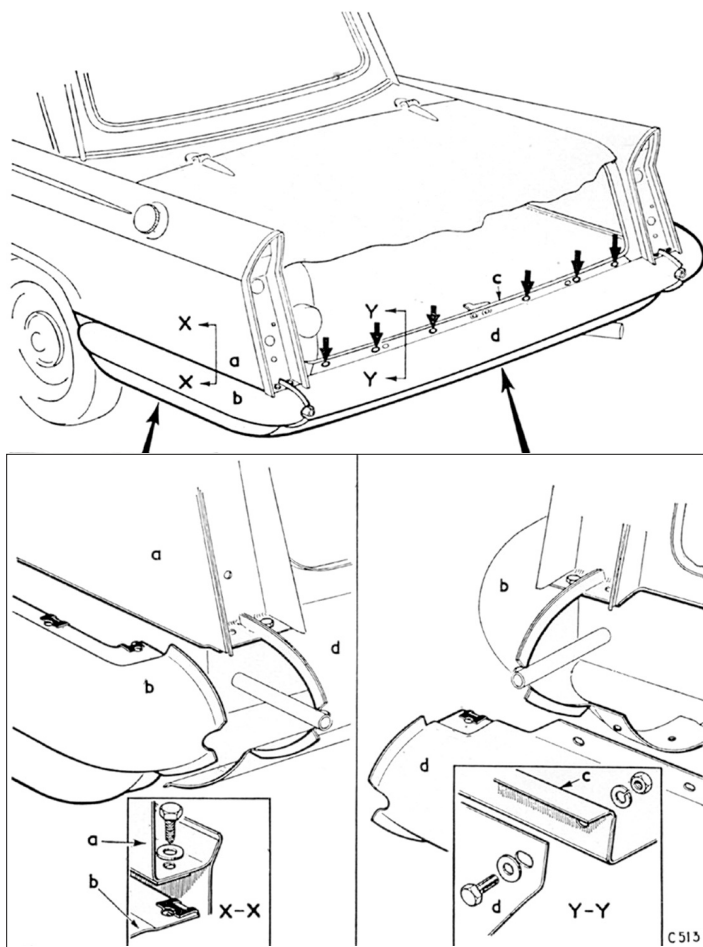
Fig. 21. Fixations des jupes latérales et arrière
