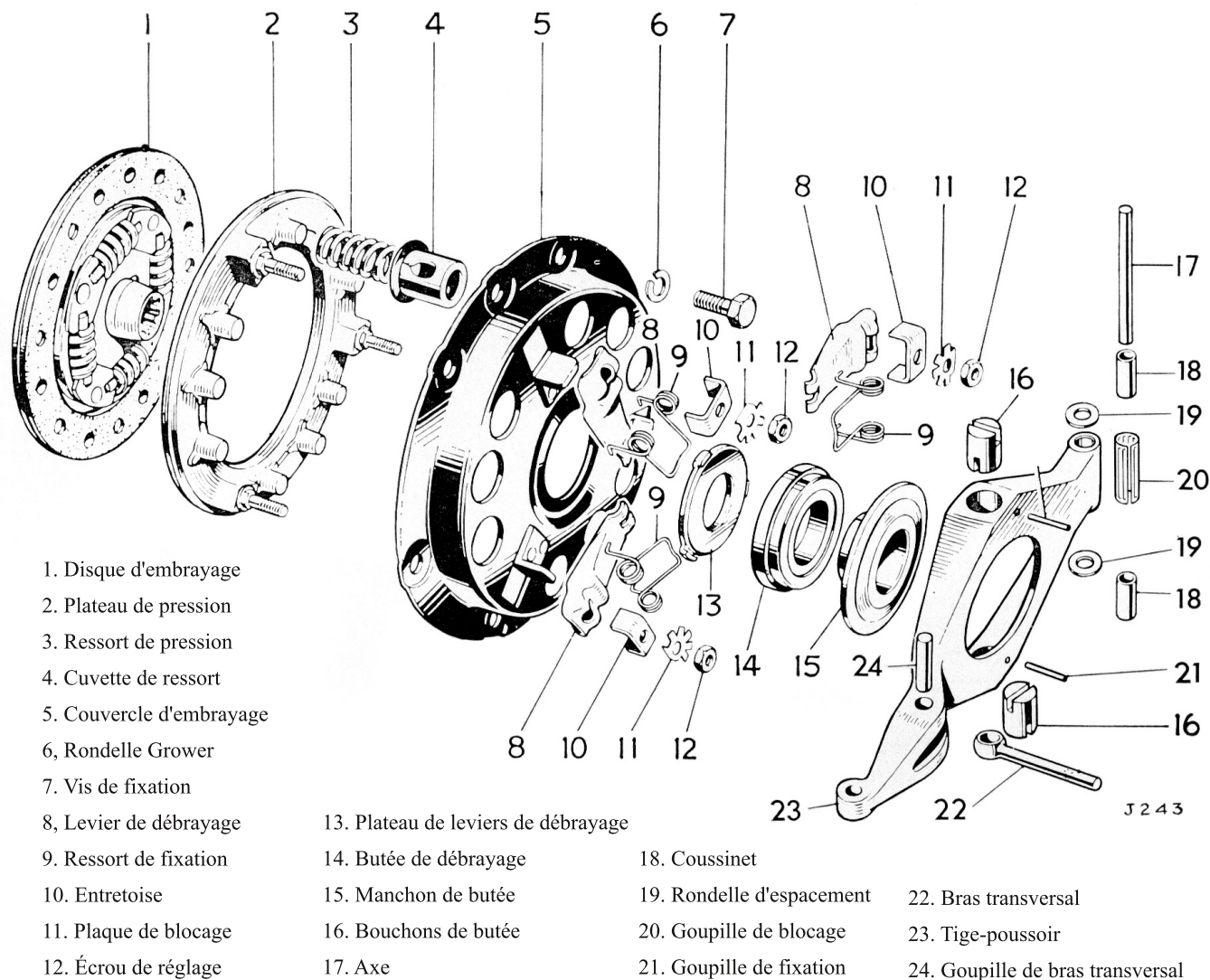
Fig. 13. Vue éclatée du mécanisme d'embrayage (Herald 1200, 12/50 et Spitfire, modèle sans diaphragme)
