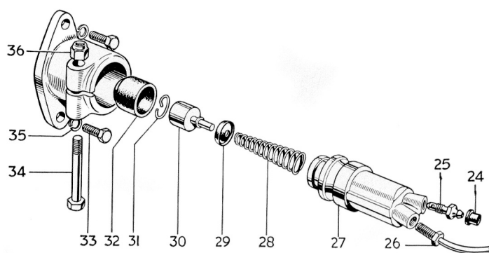
Fig. 8. Vue éclatée du cylindre de débrayage
