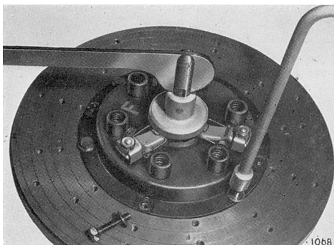
Fig. 16. Montage de l'ensemble embrayage sur l'équipement Churchill (Herald et Spitfire)
