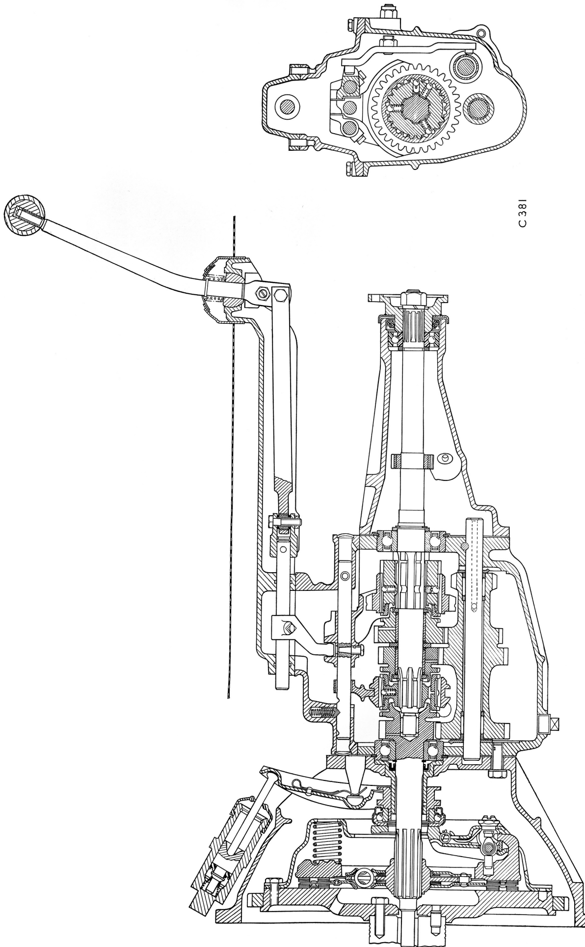
Fig. 2. Vue en coupe de l'embrayage et de la boîte de vitesses (Vitesses). La boîte de vitesses est globalement identique pour les modèles Herald 1200, 12/50, 13/60, Vitessse et Spitfire
