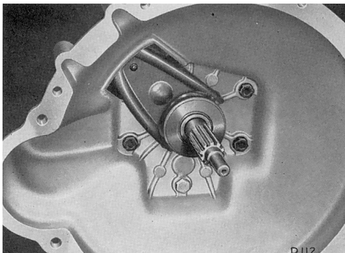
Fig. 10. Butée de débrayage (Vitesse)
