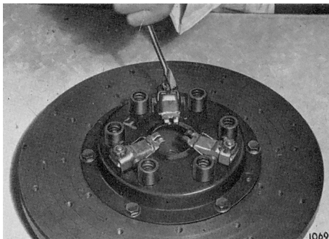
Fig. 17. Dégagement des plaques de blocage (Herald et Spitfire)
