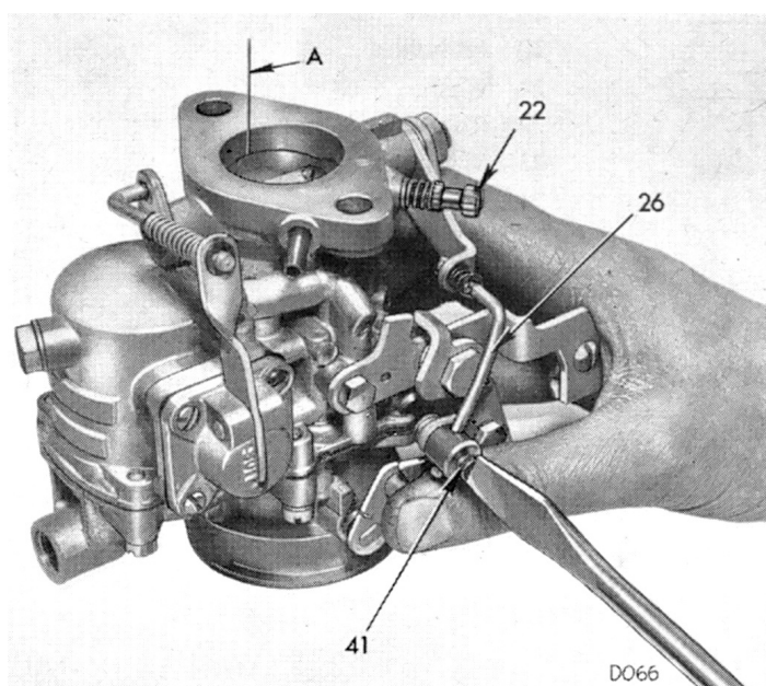
Fig. 9 : Réglage de l'interconnexion du réglage de gaz et du starter, en insérant une section de câble "A" de 0,7 mm. (0,027 ") entre le papillon et le corps du carburateur
