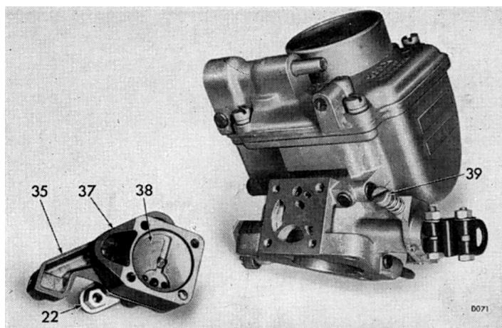
Fig. 30. Dispositif de starter détaché du carburateur
