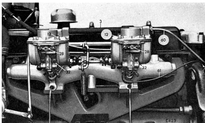
Fig. 36. Vue de droite des carburateurs
