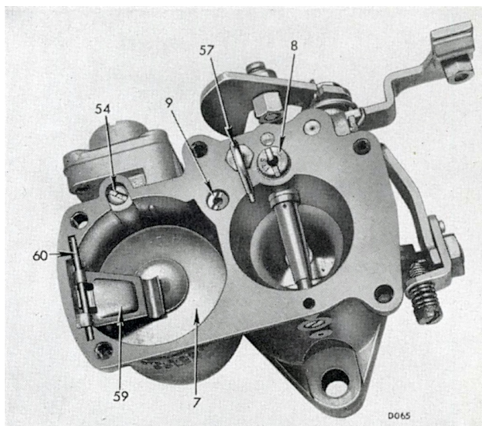
Fig. 5. Carburateur B30 PSE1 : vue interne
