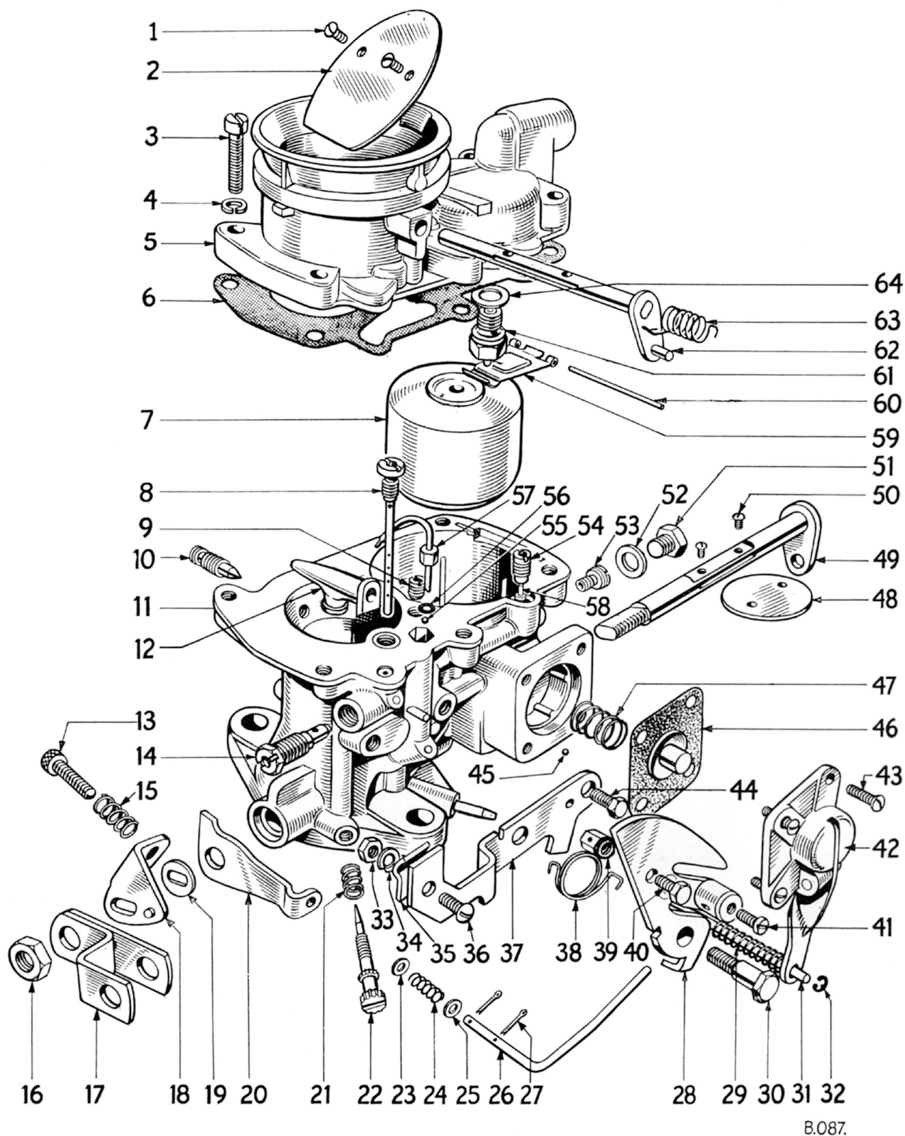
Fig. 3. Vue éclatée du carburateur Solex B30 PSE1
