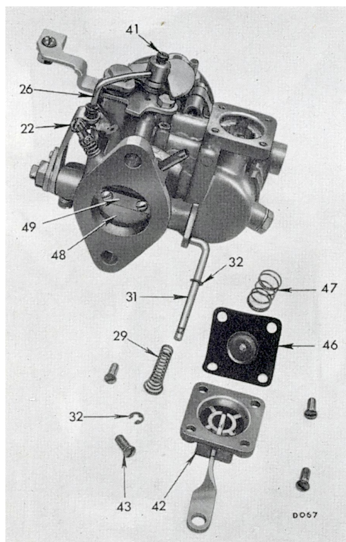
Fig. 7. Vue détaillée de la pompe de reprise
