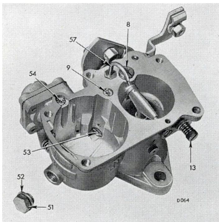
Fig. 6. Accès au gicleur principal (53) par l'orifice du bouchon (51)
