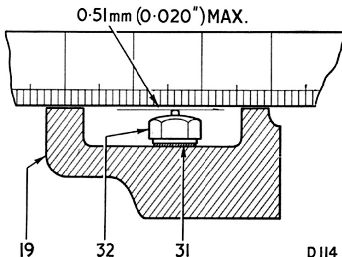
Fig. 28. Vérification de la hauteur du pointeau
