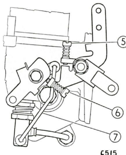
Fig. 15. Vis d'ajustage de l'interconnexion entre le gicleur et la commande de starter
