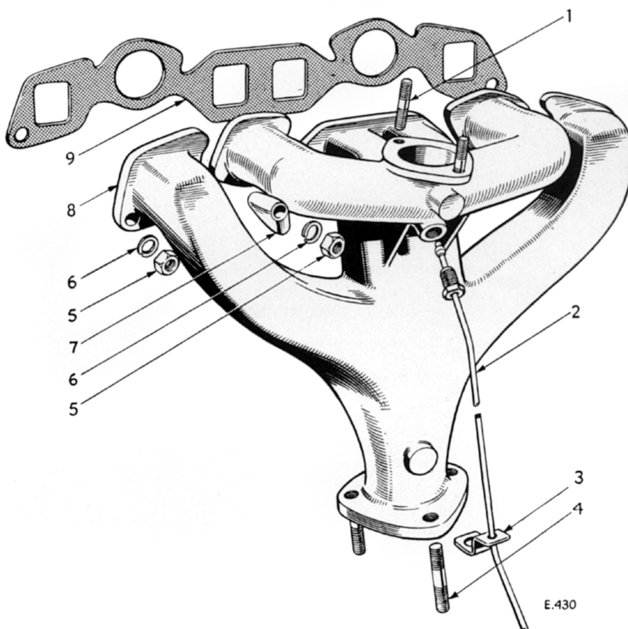
Fig. 2 Détails du collecteur - Herald 12/50
