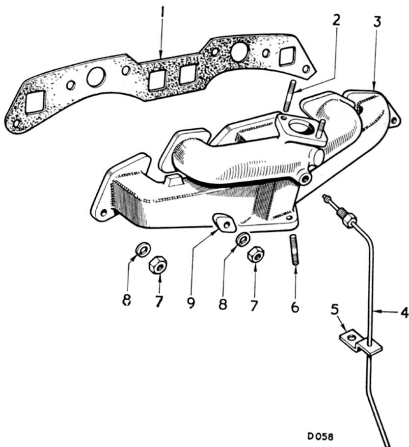
Fig. 1 Détails du collecteur - Herald 1200
