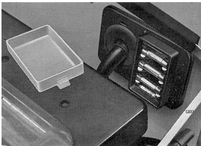
Fig. 9. Boîtier de fusibles
